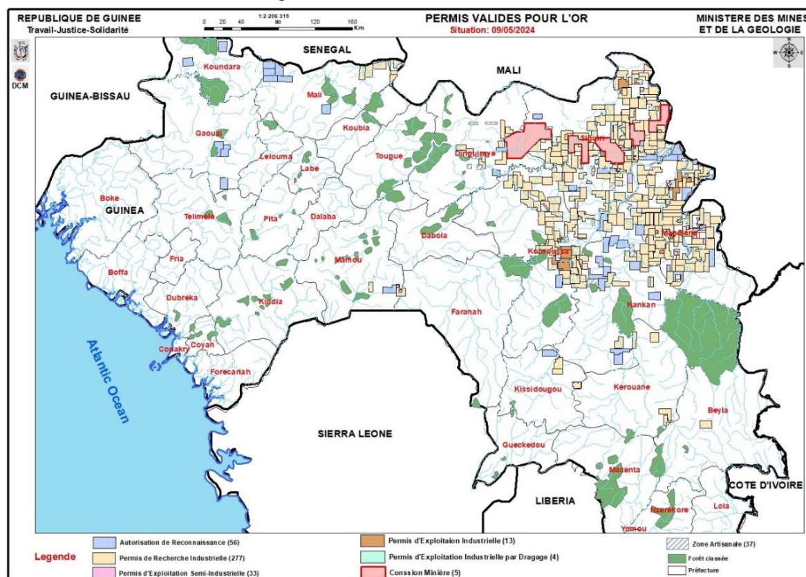
Figure 10 : carte des ressources en or
