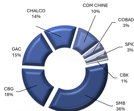
Figure 17: Production de bauxite par société
