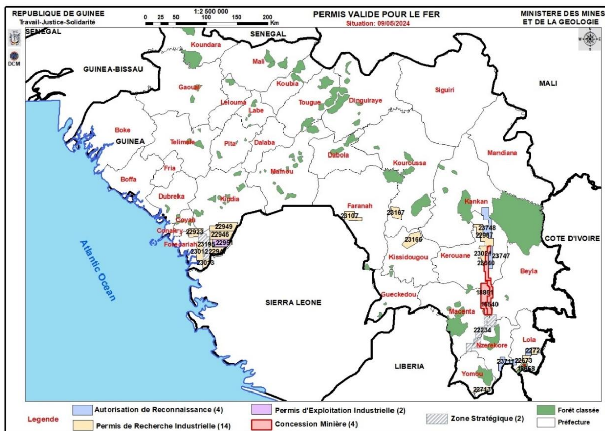
Figure 9 : Principaux gisements pour le Fer
