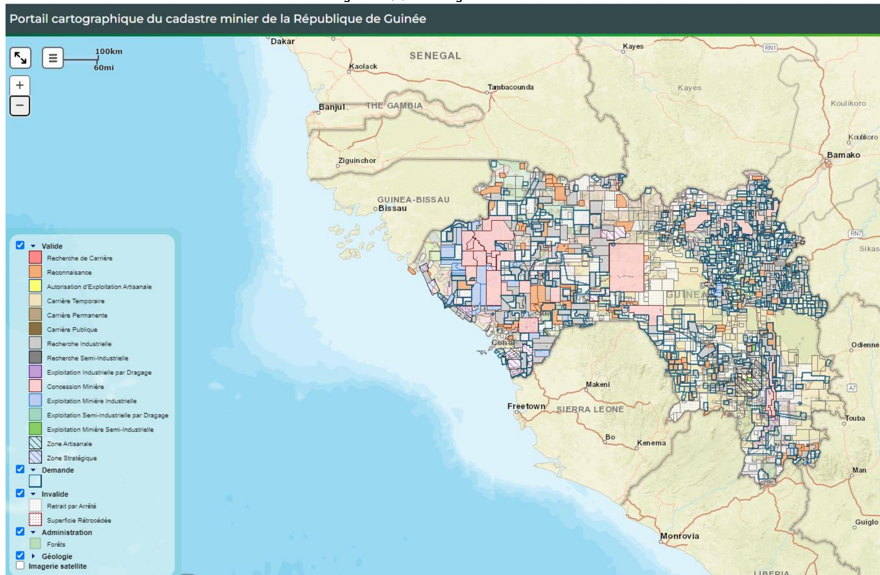
Figure 15 : Carte des gisements des titres miniers
