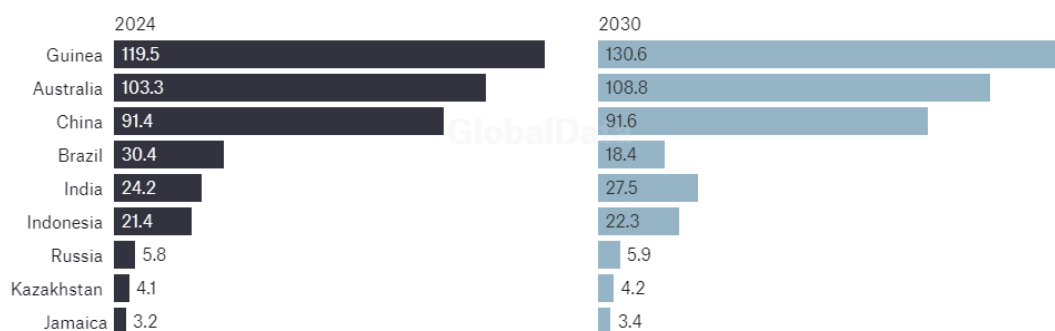
Figure 8 : Estimation de la production de bauxite pour 2024 et 2030 12
