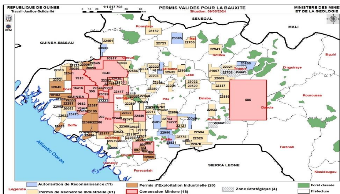
Figure 6 : Permis Valide pour la Bauxite
